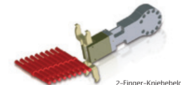
2-Finger-Kniehebelgreifer für die Beladung von Wellenteilen
