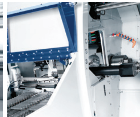
Vollautomatische Beladung von Wellen. Zuführung über Taktband, Abführung über die Fertigteilaufrangvorrichtung.
