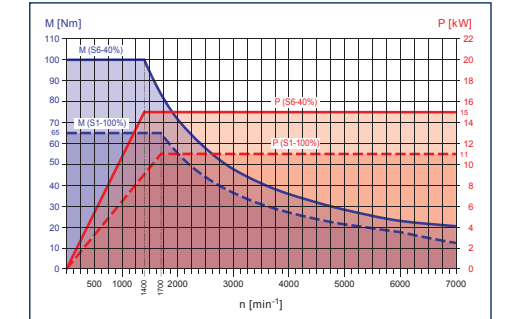
HYPERTURN 45-G3 Hauptspindel/Gegenspindel
